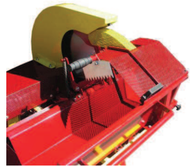
Griffeinrichtung zum Fixieren des Schnittgutes
